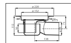
SIPHON PURUS ODEN réf. 1416 003 Débit 3L/s
