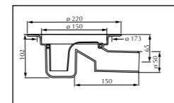
SIPHON PURUS FREJA réf. 1416 002 Débit 2L/s
