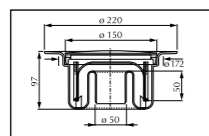
SIPHON PURUS DUSCHBRUNN réf. 1416 001 Débit 2L/s
