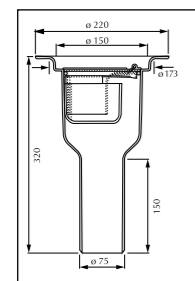
SIPHON PURUS BRAGE 75 réf. 1416 005 Débit 3L/s
